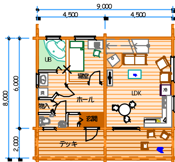
一階平面プラン 16.4坪)
