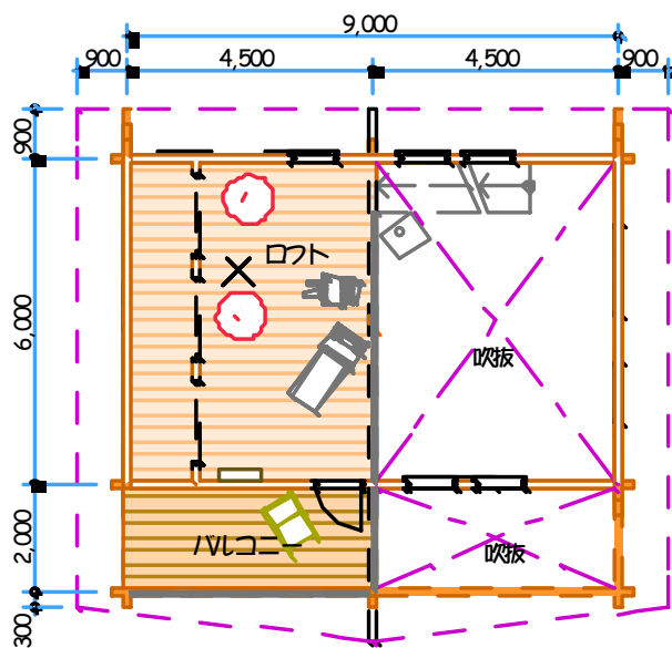
ロフト平面プラン 27.0㎡ (8.2坪)
