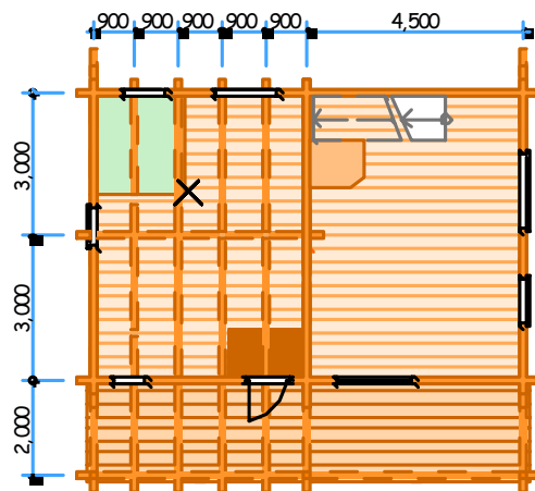
ロフト根太配置図
